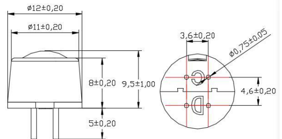
图 1：传感器外形结构图
