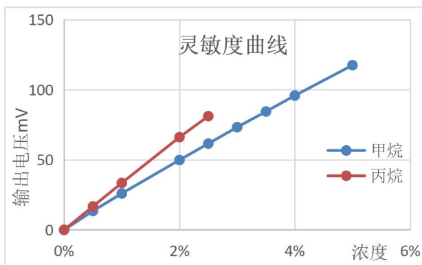
图 3: 灵敏度特性曲线
