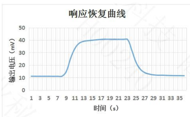
图 4: 响应恢复特性曲线
