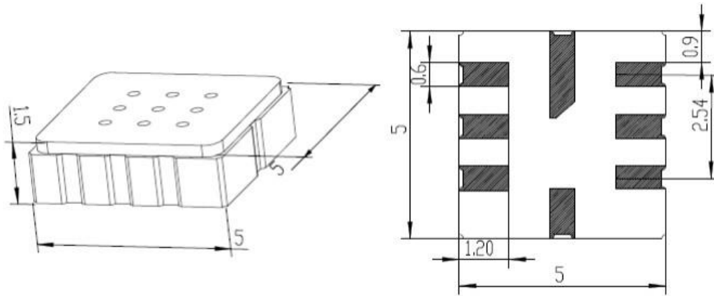
图 2: ZM03 尺寸图
