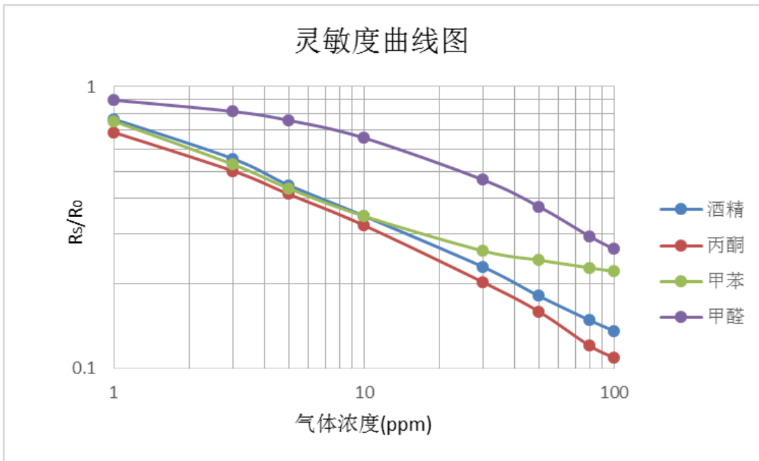
图 3: 灵敏度曲线
