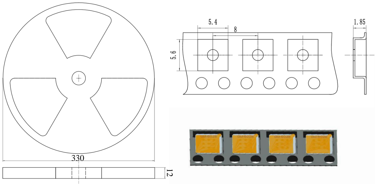
模组包装图
