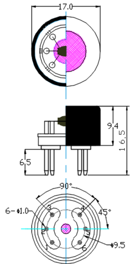
图1 传感器结构图
