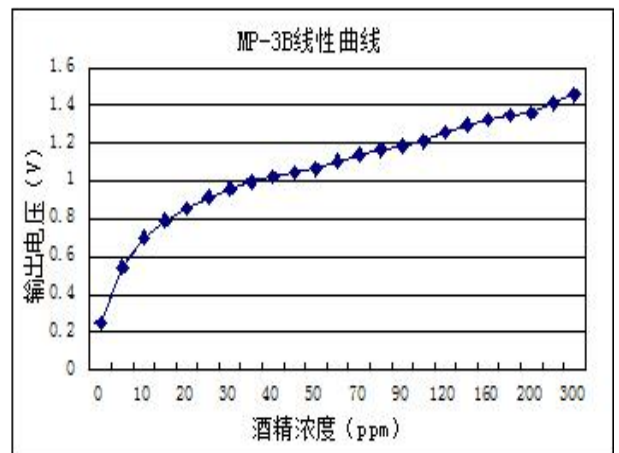
图6：传感器线性曲线
