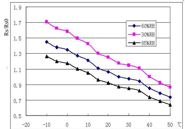
图4：传感器典型的温度、湿度特性曲线
