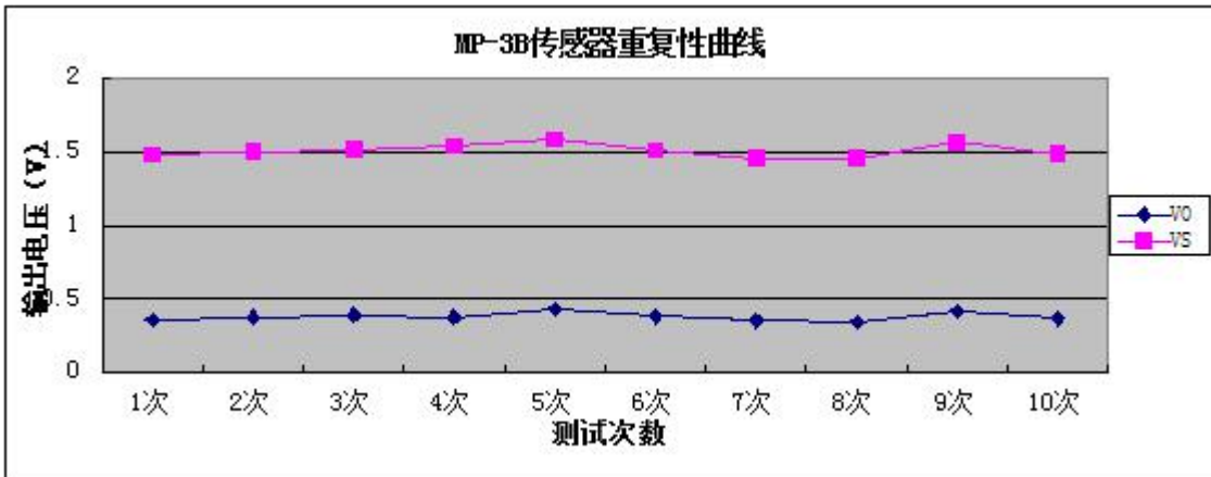
图 7: 重复性曲线
