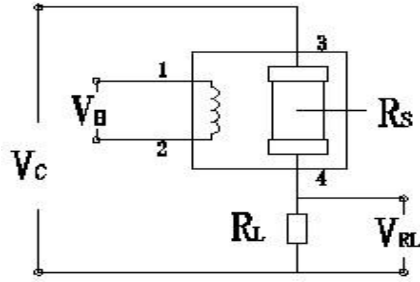
图2：MP-3B 测试电路
