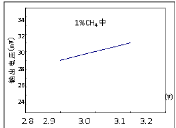
图 10：灵敏度电源波动特性曲线
