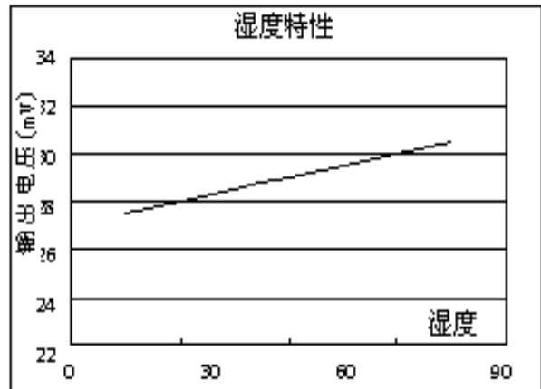
图 8: 灵敏度湿度特性曲线
