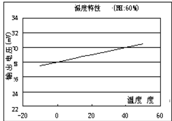
图 6: 灵敏度温度特性曲线
