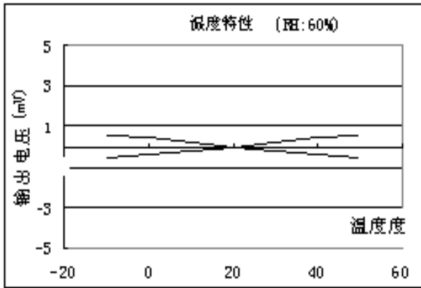
图 5: 零点温度特性曲线
