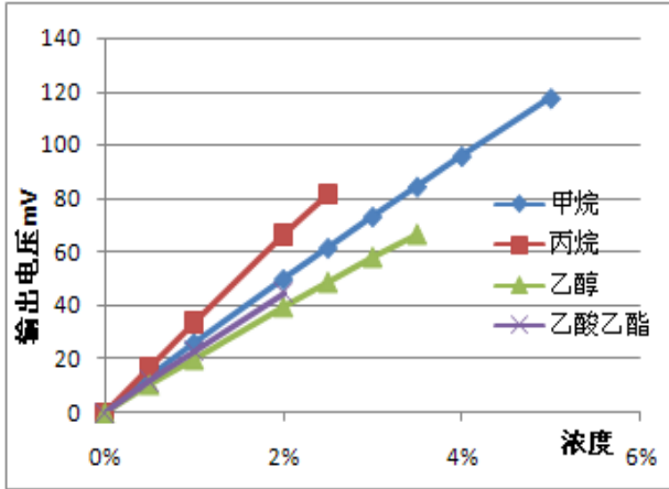
图 3: 灵敏度曲线
