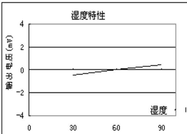
图 7: 零点湿度特性曲线
