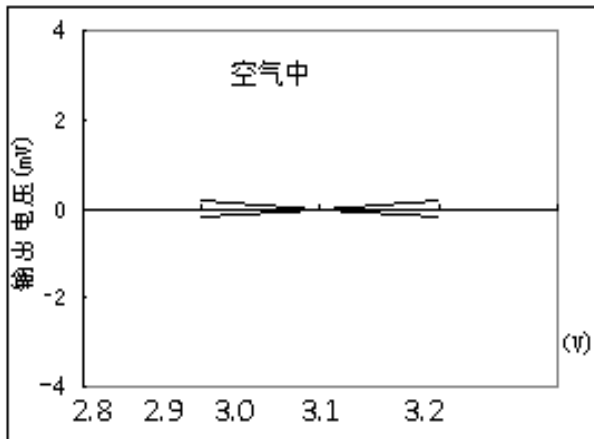
图 9：零点电源波动特性曲线
