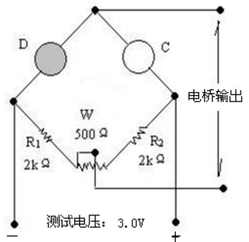
图 2：基本测试电路
