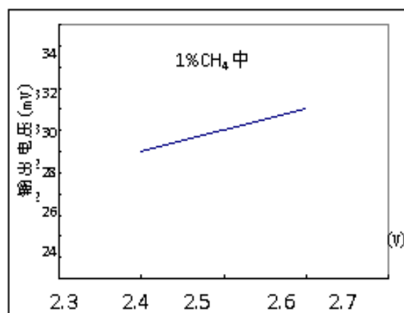
图 10：灵敏度电源波动特性曲线
