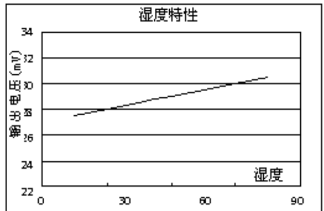
图 8: 灵敏度湿度特性曲线
