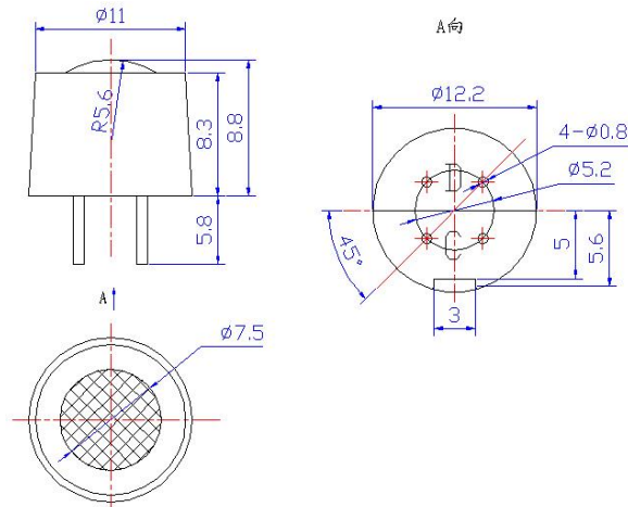
图 1：元件外形结构图
