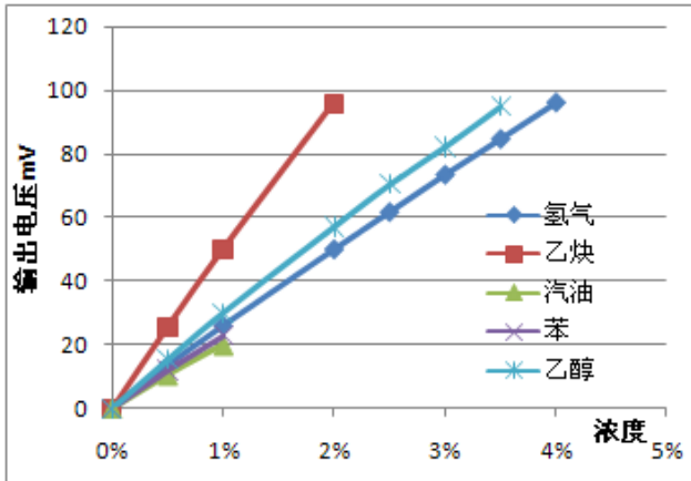
图 3: 灵敏度曲线
